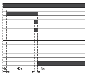
Vypnutí kvůli poruše zapálení (A)
