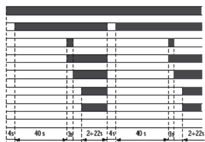
Omezený počet pokusů o restart (B)
