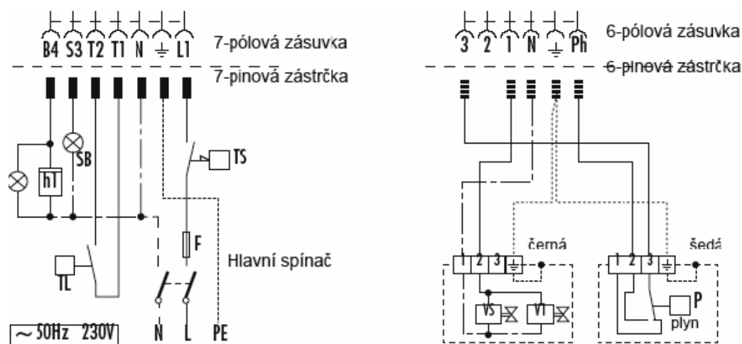
Automatika se zapalovacím transformátorem
