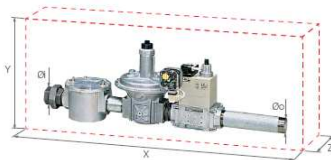
Příklad plynové řady typu COMPOSED bez kontroly těsnosti
